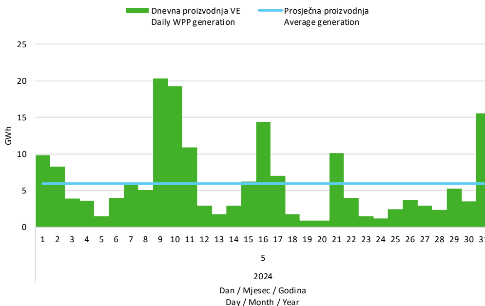
Slika 5 Dnevna proizvodnja svih vjetroelektrana u svibnju 2024. godine
